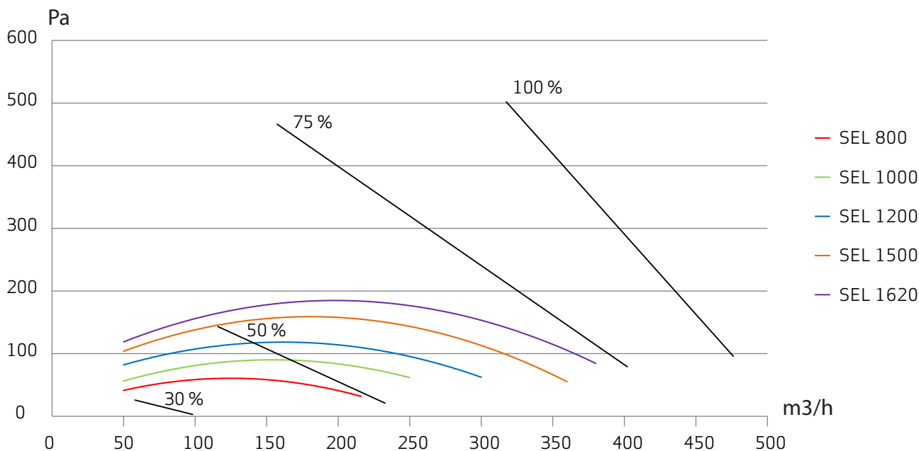
Premium Preheat 250 XL SEL-faktorer målt iht. EN13141-7 (ALU: Coarse/ePM1)
